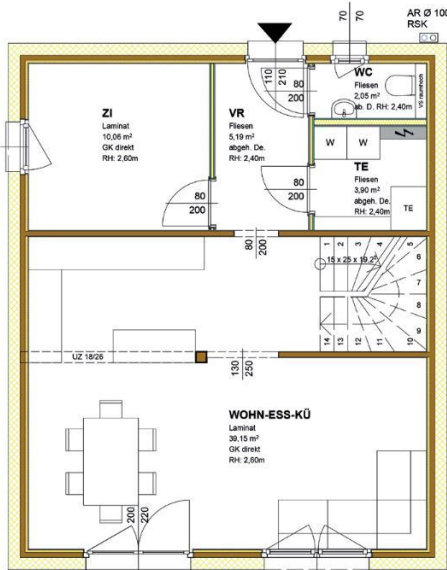
Grundriss Erdgeschoß
