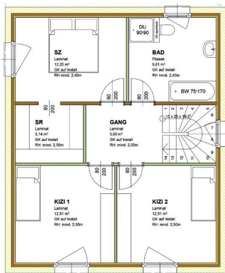
Grundriss Obergeschoß
